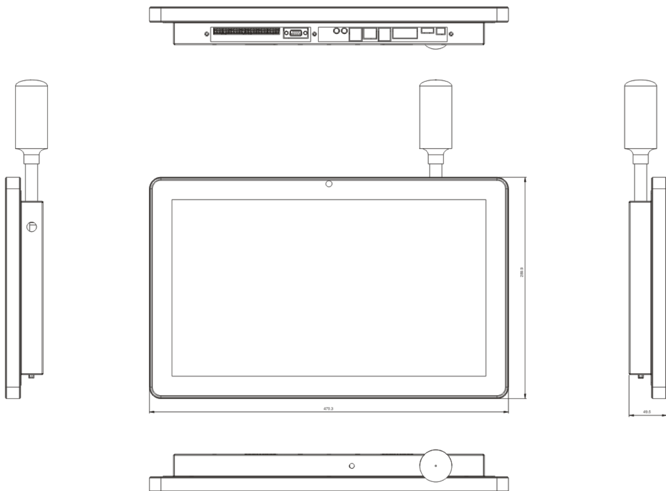
图2.1 18.5寸产品正面侧面尺寸图
